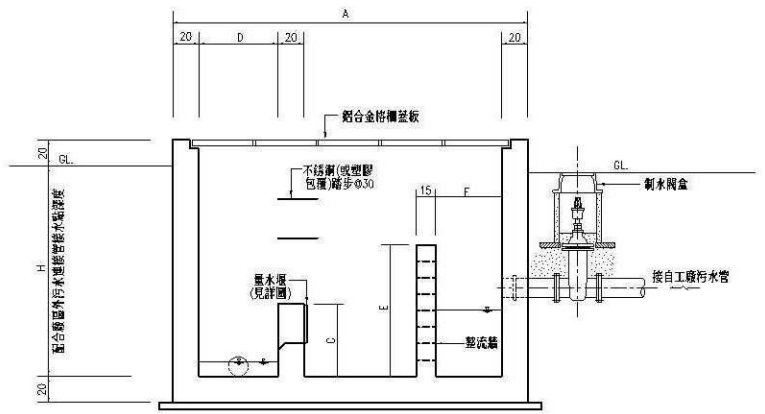
剖面圖
