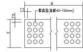
整流牆開孔示意圖
